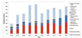
图1-1 2004-2013年核电厂因自然灾害导致的停机小时数
